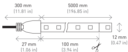
IP68 72W RGB (60 LEDs/m)
