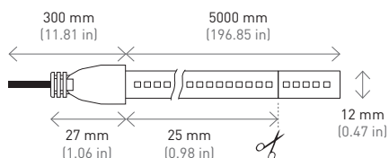
IP67 84W (240 LEDs/m)
