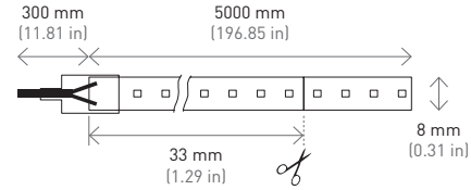
IP20 72W (180 LEDs/m)
