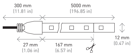
IP67 43W (36 LEDs/m)
