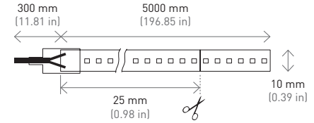
IP20 84W (240 LEDs/m)
