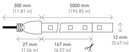
IP67 43W (36 LEDs/m)
