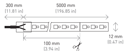
IP20 80W RGBW (120 LEDs/m)
