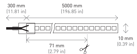
IP20 84W (84 LEDs/m)
